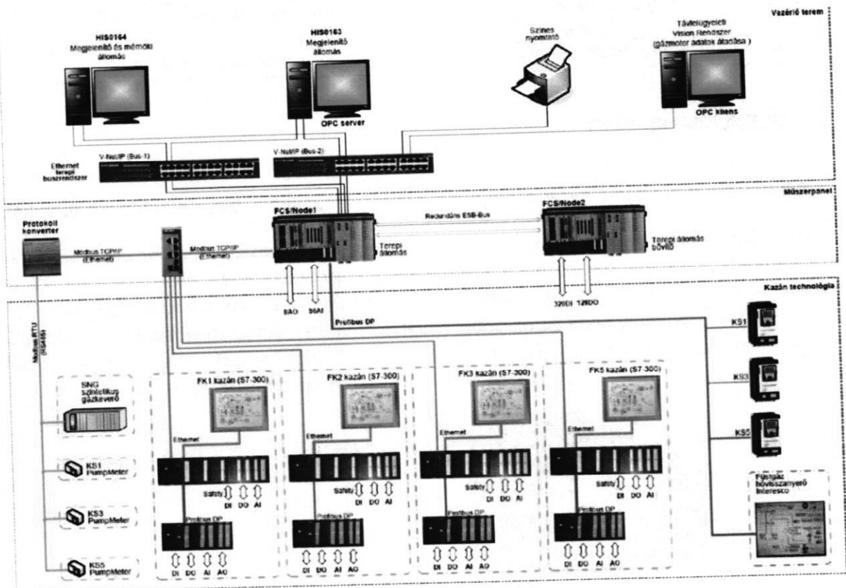
2. ábra - jelenlegi folyamatirányító rendszer sémarajza
