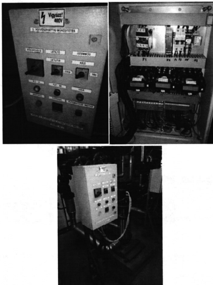
7. ábra - Pótvízszivattyú meglévő kapcsolószekrénye
