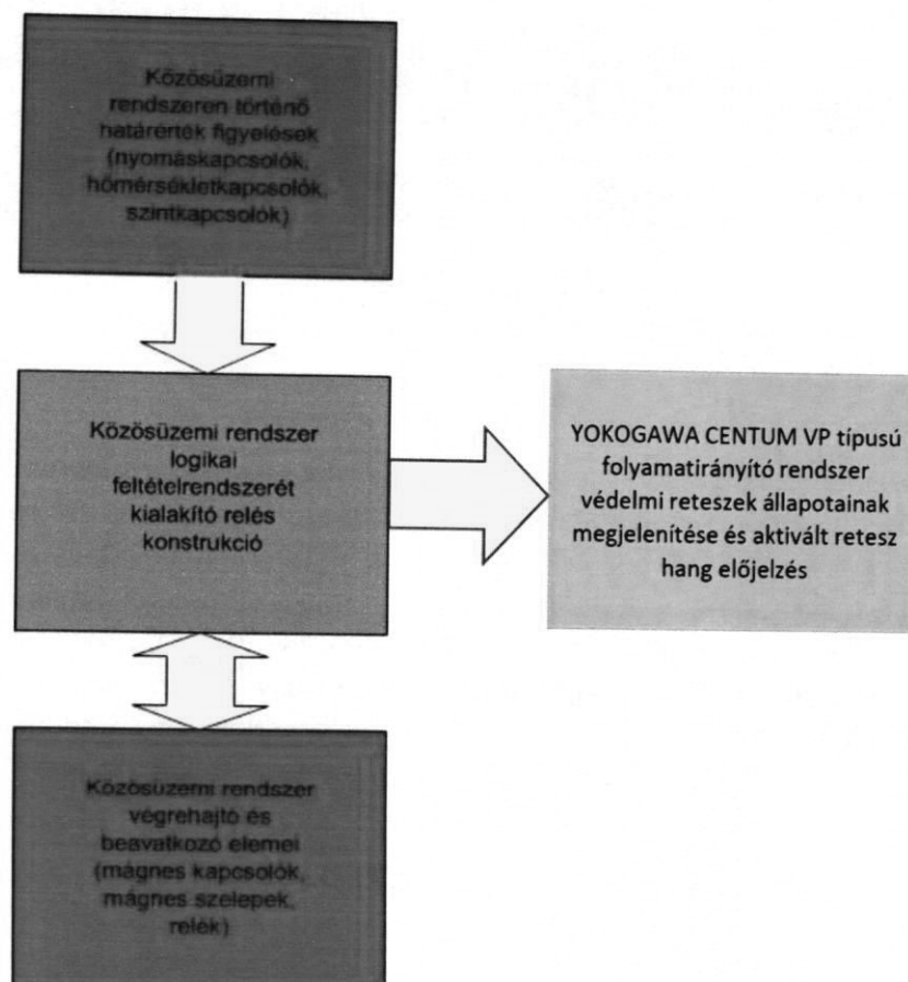
1. ábra – jelenlegi felépítés
