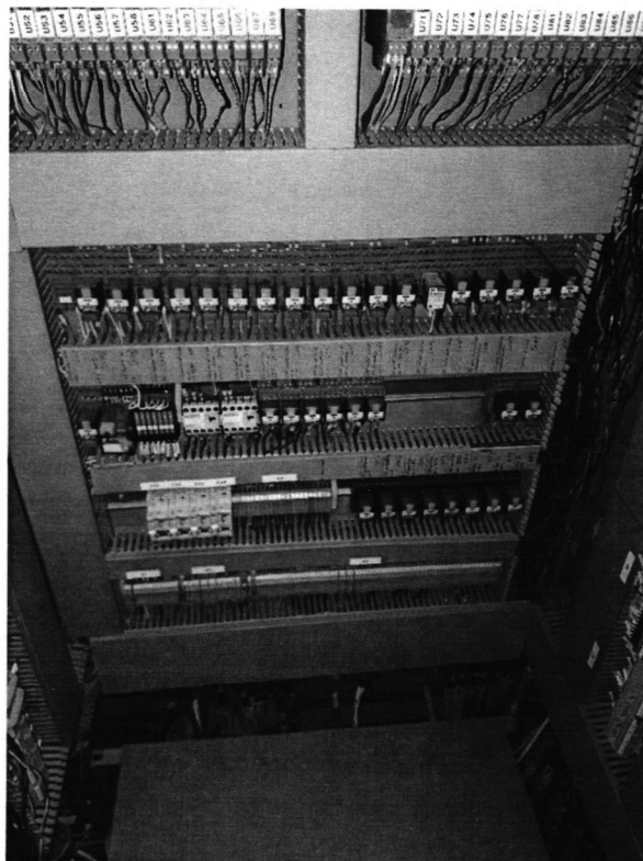
3. ábra – Közösüzemi relé rendszer
