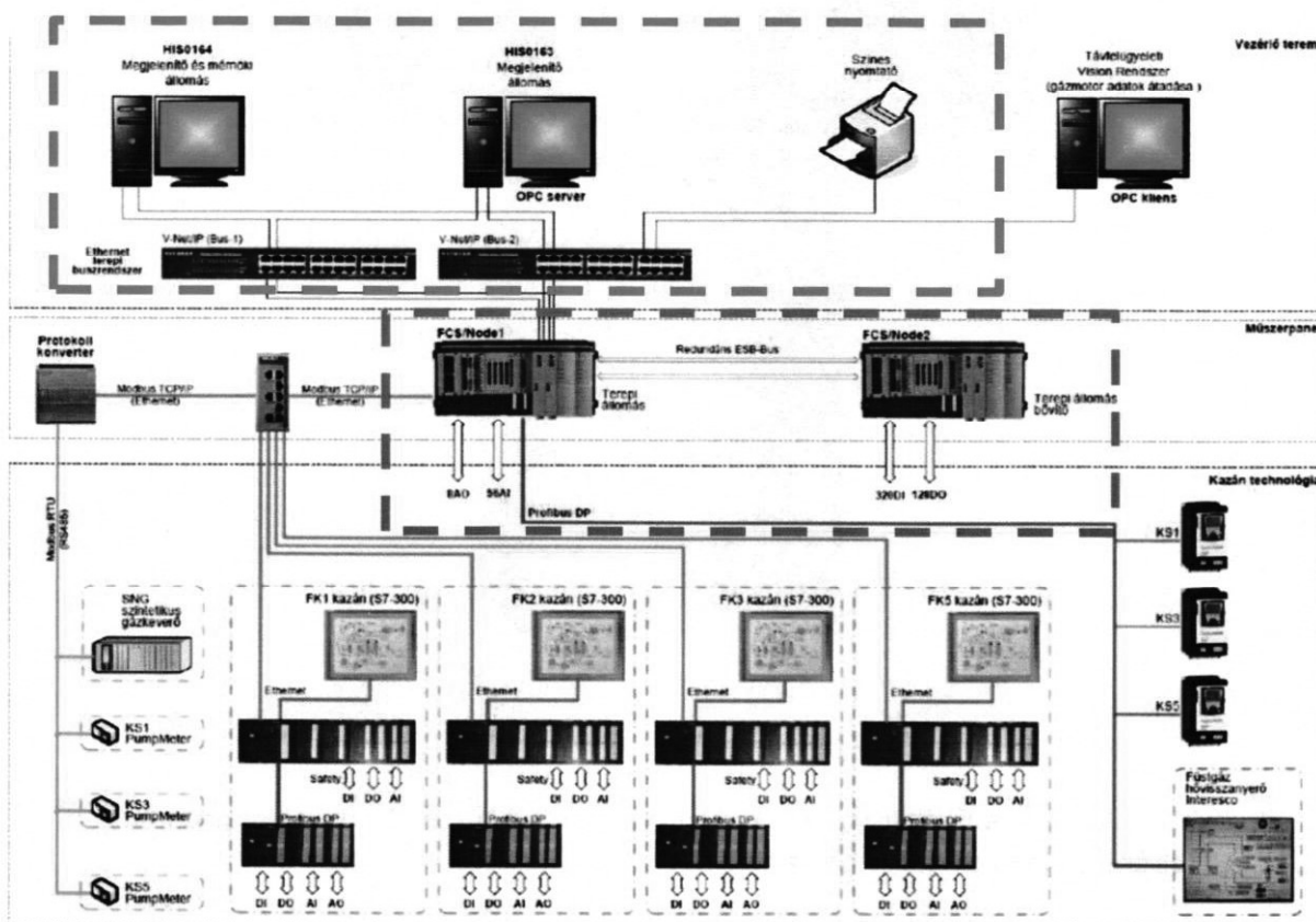
6. ábra - jelenlegi folyamatirányító rendszer cserélendő eszközök
