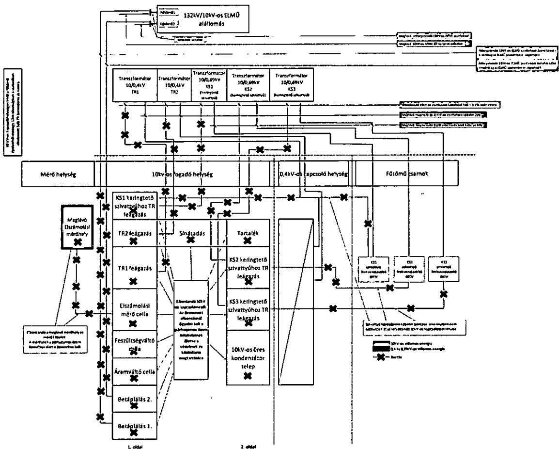
5. ábra: 10kV-os kapcsolószekrény és kábelek bontási rajza
