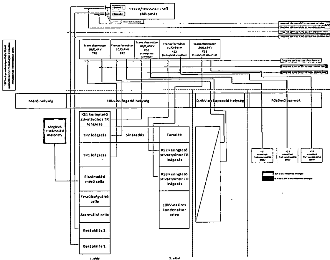
1. ábra: 10 kV-os helyiség és kábelösszefüggés jelenlegi felépítése
