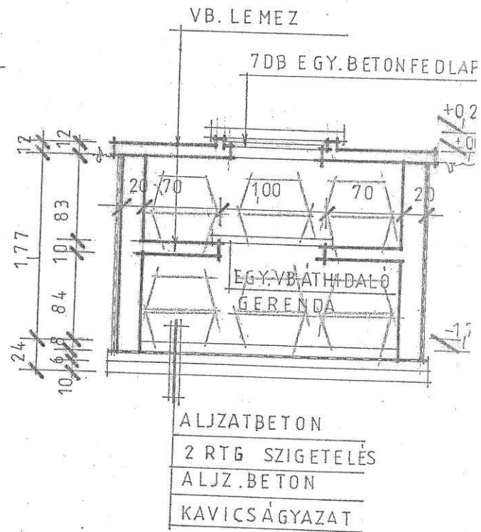
A-A METSZET
