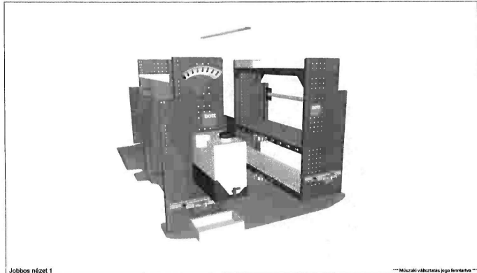
Jobbos nézet 1
